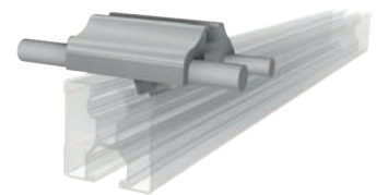
Morsetto parafulmini superiore, altezza d'ingombro molto ridotta per moduli con telaio di 30 mm altezza
